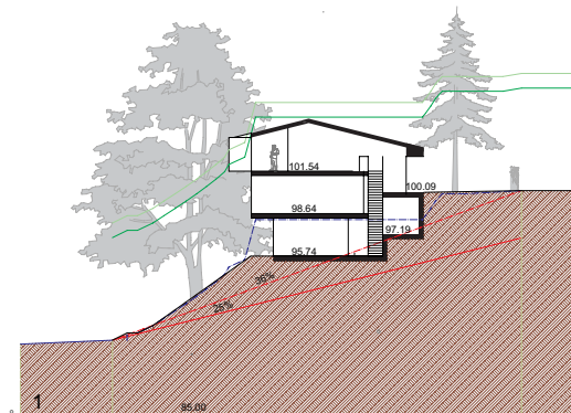
coupe générale
